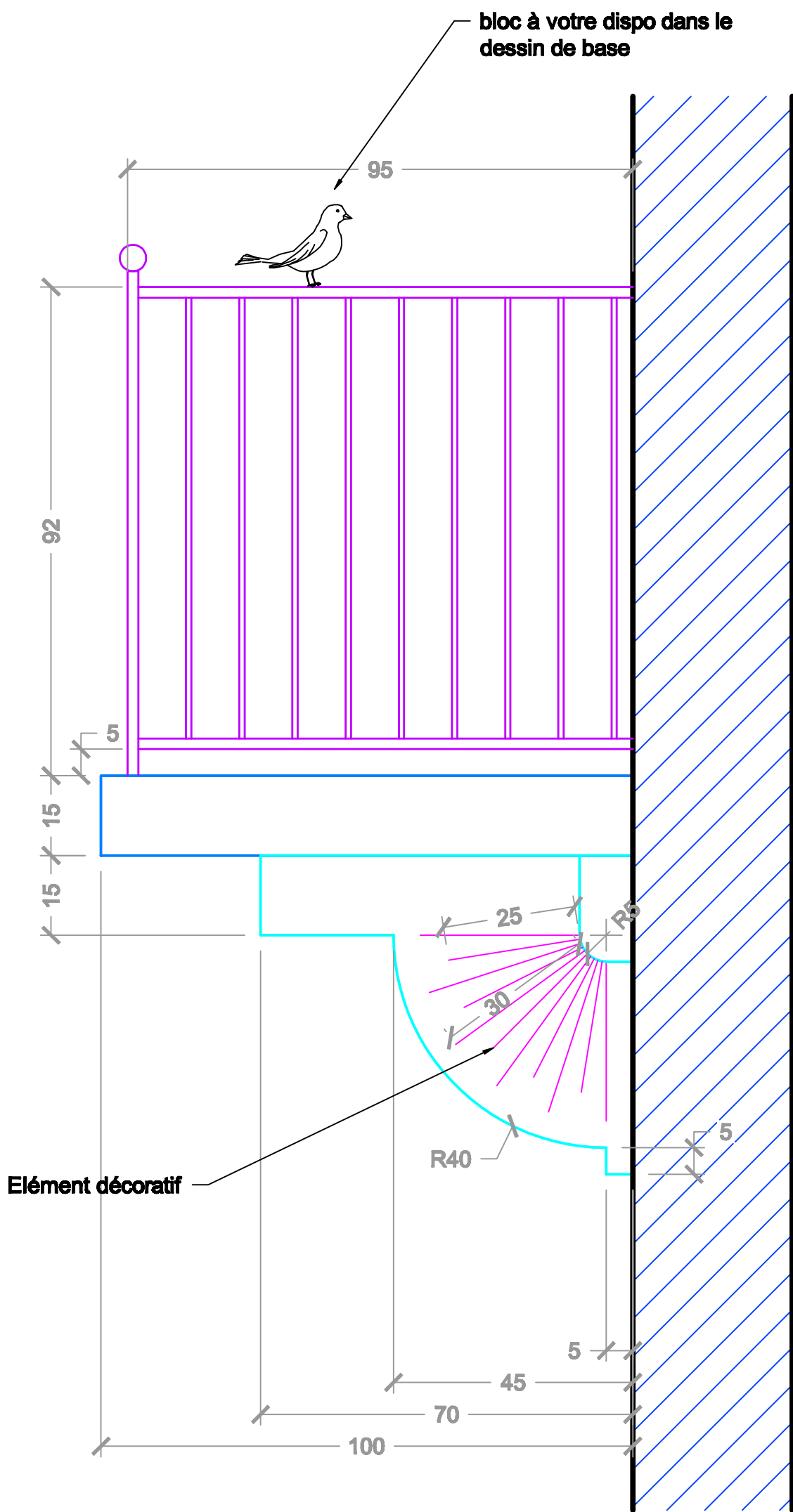
profil balcon 1:10
