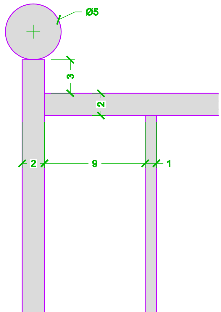
détail garde corps 1:2
