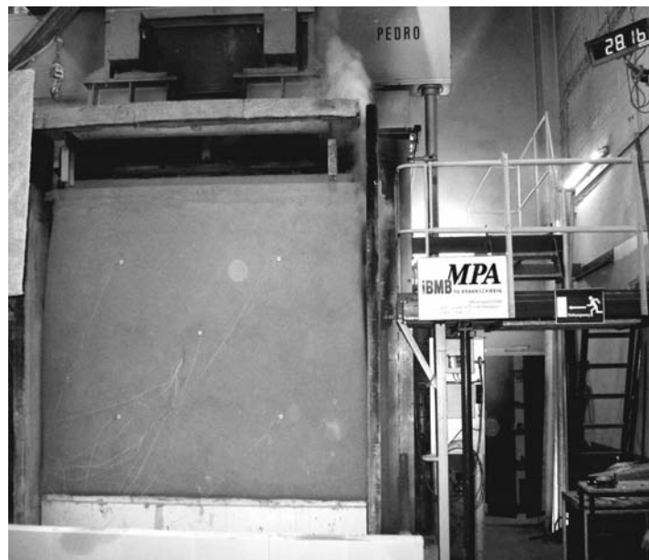
Test de résistance au feu allemand (2003)
