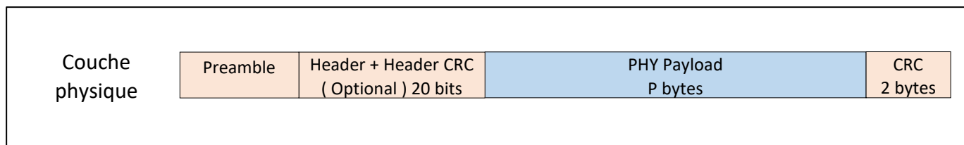
Figure 94: Détail de la couche physique LoRa
