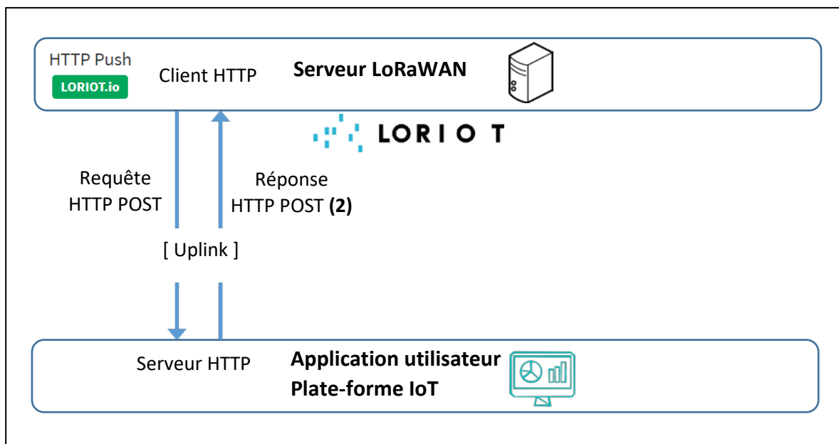
Figure 114: Uplink HTTP POST avec LORIENT
