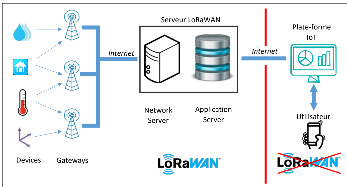
Figure 30: Architecture globale d'un réseau LoRaWAN
