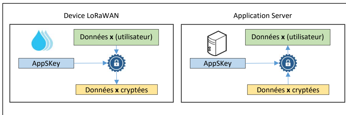
Figure 38: Processus de chiffrement et de déchiffrement
