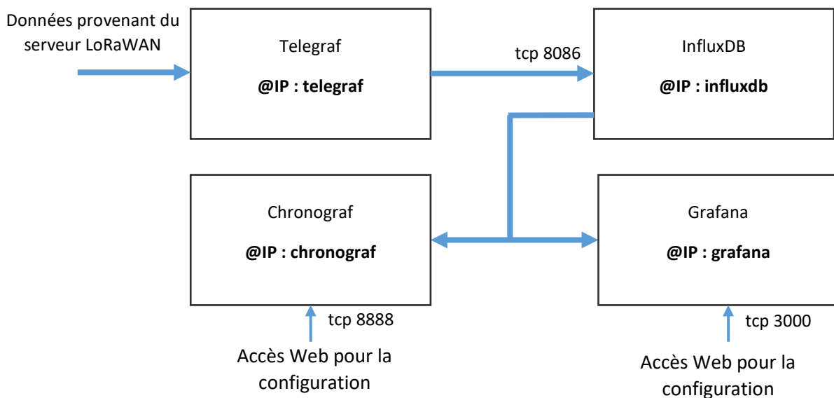
Figure 154: Conteneurs Docker pour notre application utilisateur
