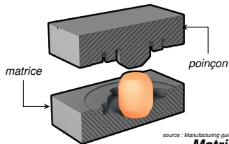
Matriçage
