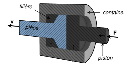
Extrusion simple
