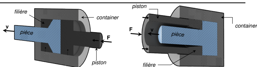
Extrusion directe
