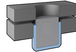
emboutissage
