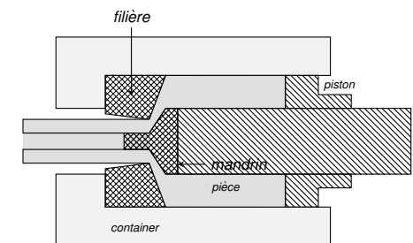
Mandrin fixe
