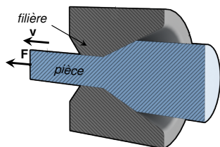
Tréfilage simple
