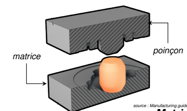
Matriçage
